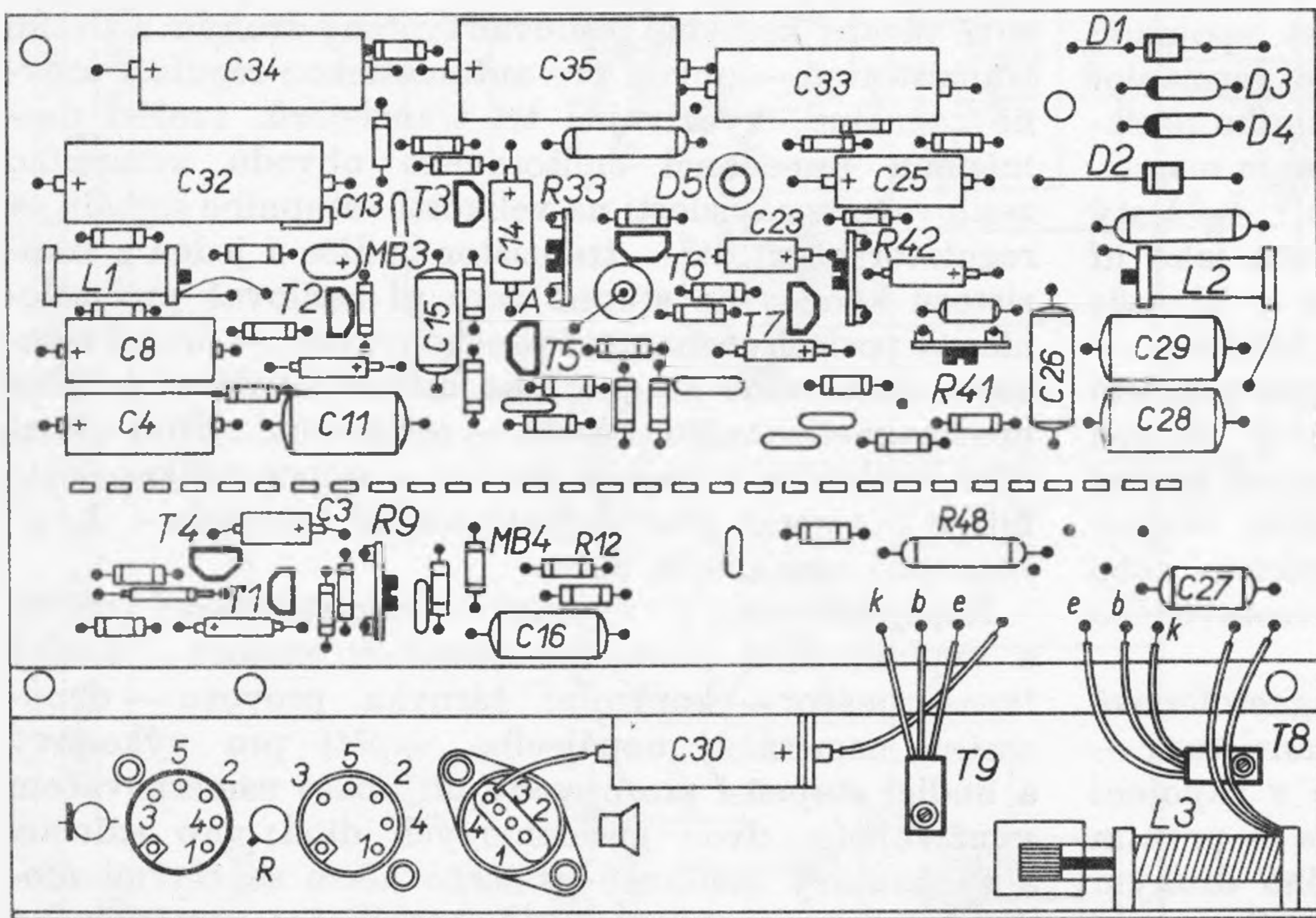
Rozmístění nastavovacích prvků na desce magnetofonové části
