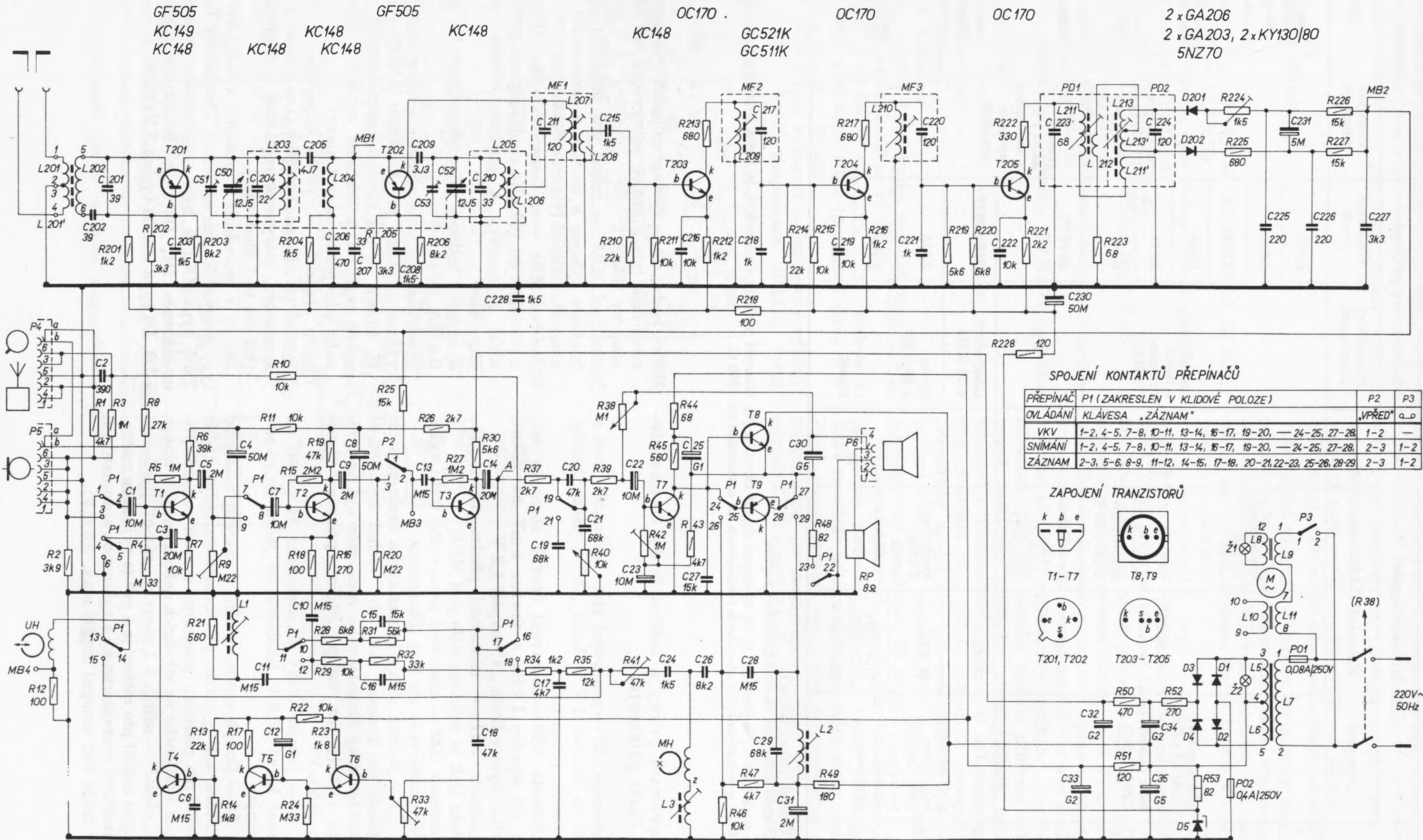
Zapojení přijímače s magnetofonem ANP 284 „B200“
