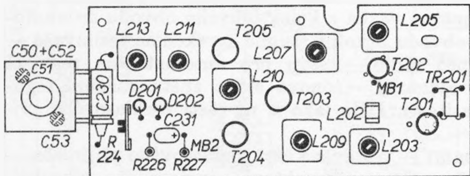
Rozmístění sladovacích prvků na desce přijímače
